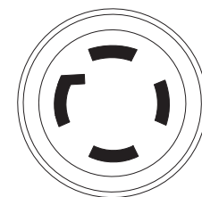
Figura 12 - Receptáculo de 120/240 VAC, 30 Amp
